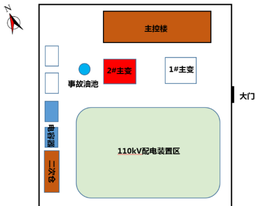
图 2 高坪 110kV 变电站总平面布置示意
