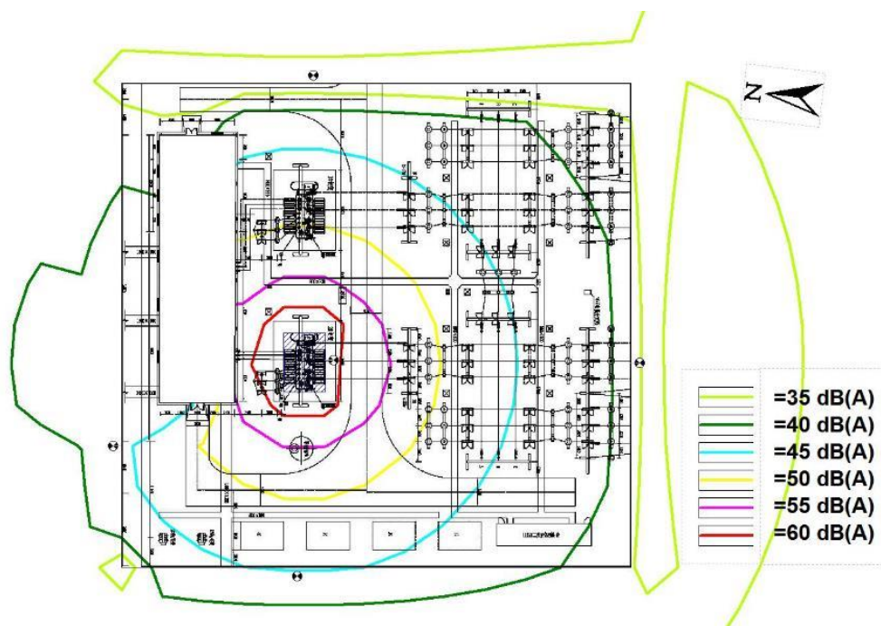
图 10 高坪 110kV 变电站本期规模噪声预测等值线图
