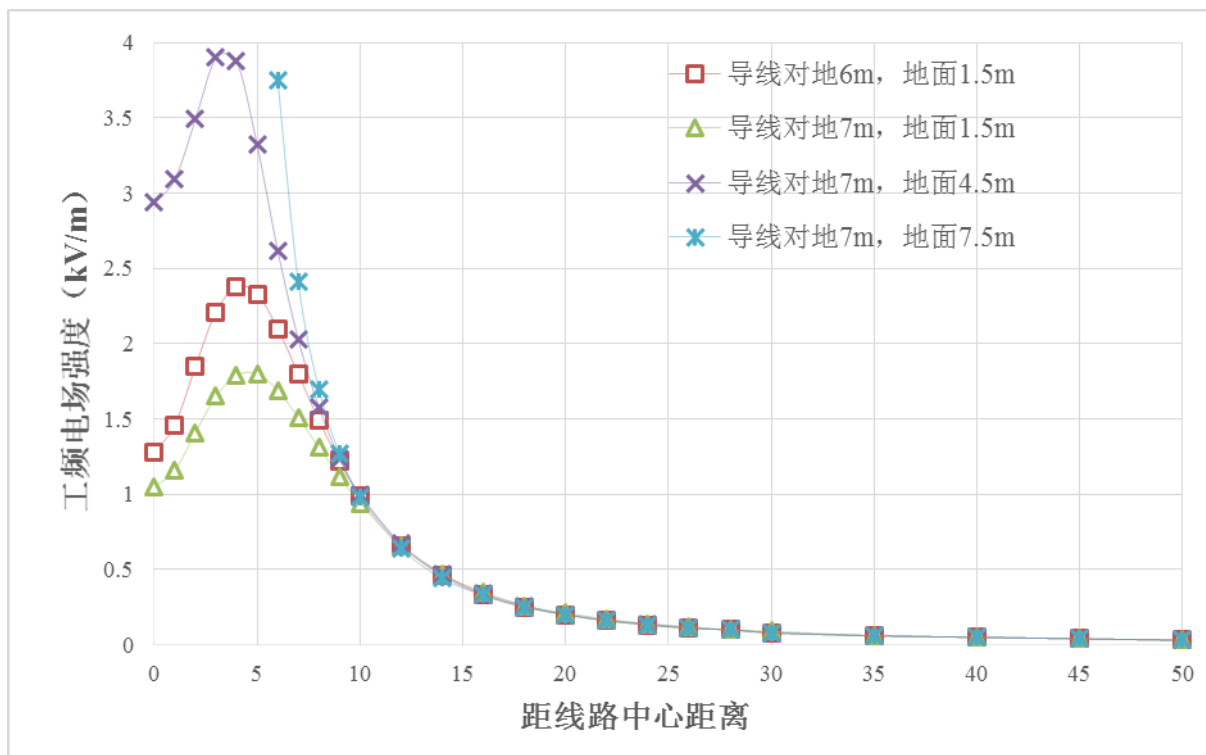
图 14 110kV 单回线路工频电场预测分布图
