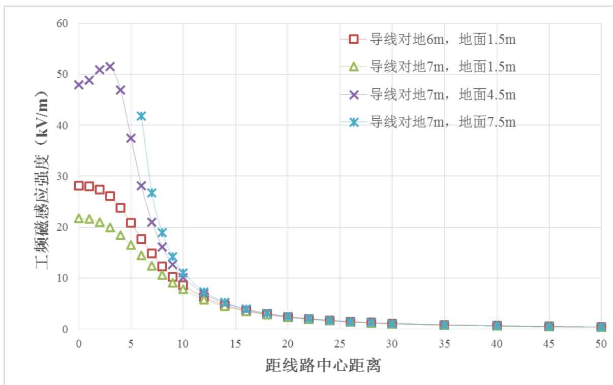
图 15 110kV 单回线路工频磁场预测分布图
