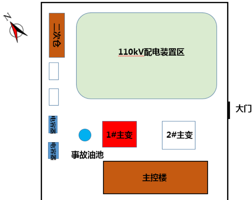
图 2 五峰铺 110kV 变电站总平面布置示意
