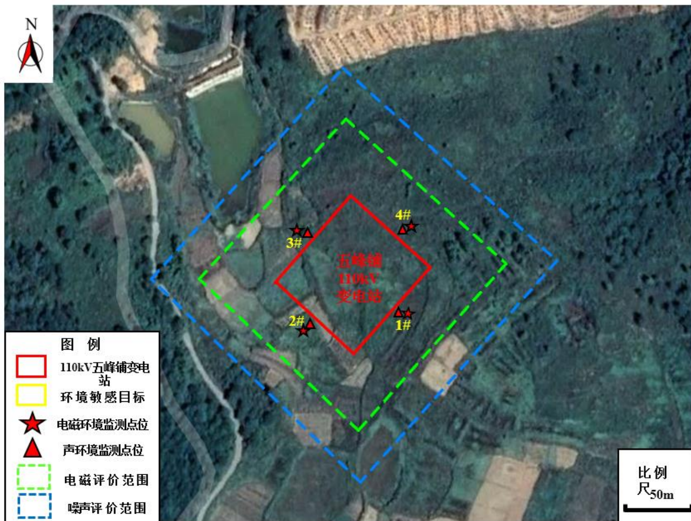
图 5 五峰铺 110kV 变电站周围敏感点相对位置关系示意
