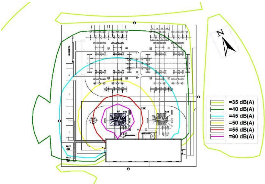
图 10 五峰铺 110kV 变电站本期规模噪声预测等值线图
