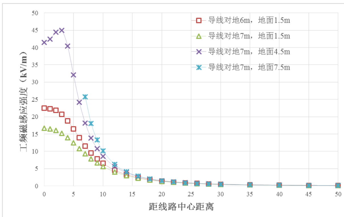
图 17 110kV 双回线路工频磁场预测分布图
