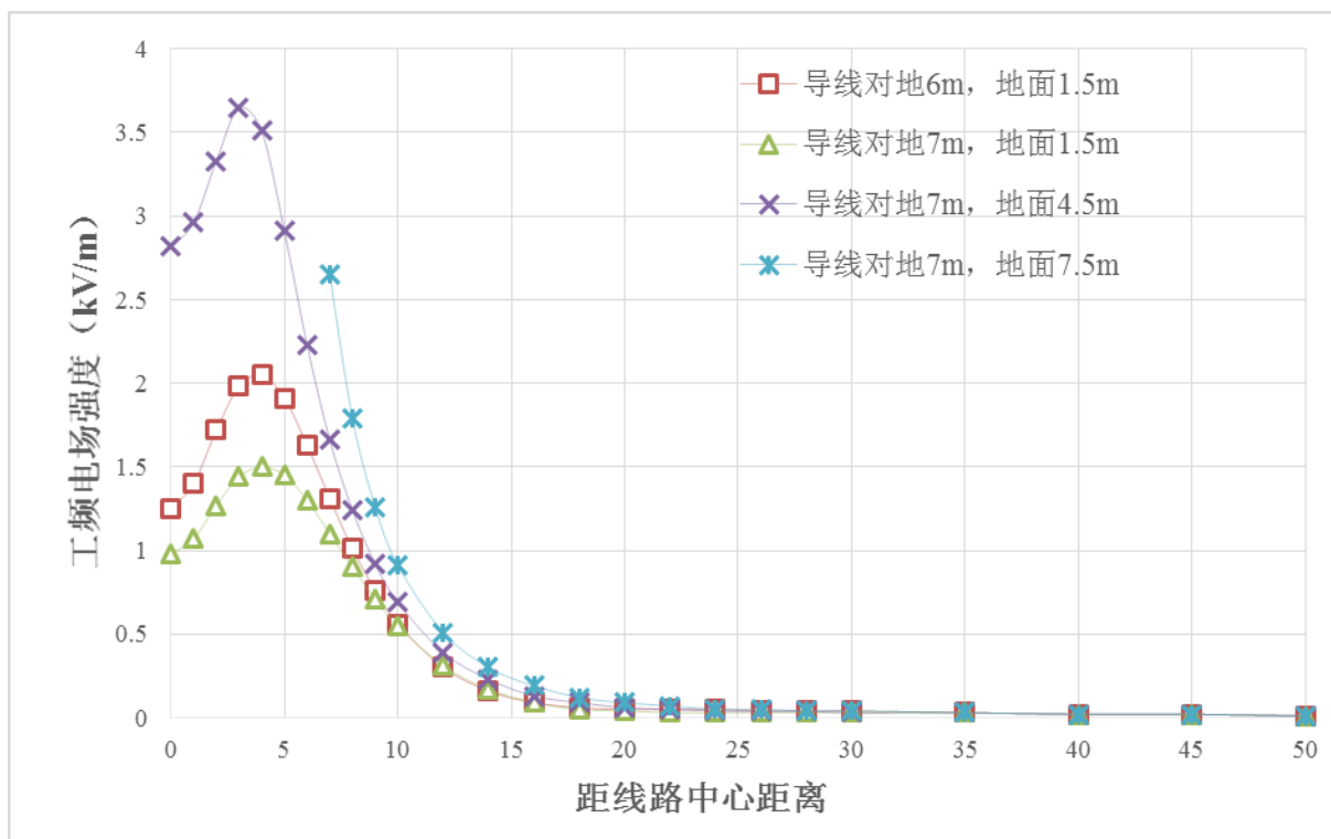
图 16 110kV 双回线路工频电场预测分布图
