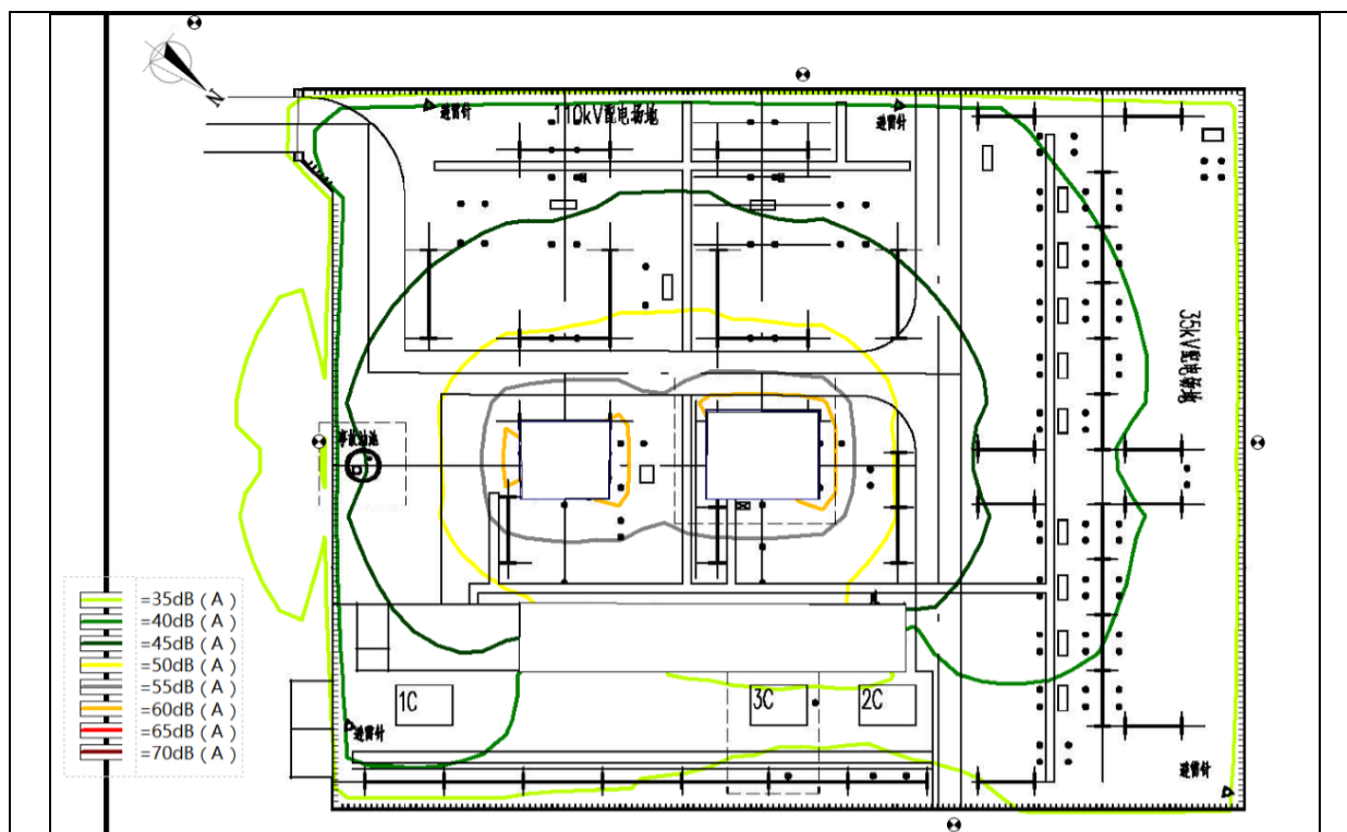
图 9 浦口 110kV 变电站本期规模噪声预测等值线图(按照终期 2 台主变预测)
