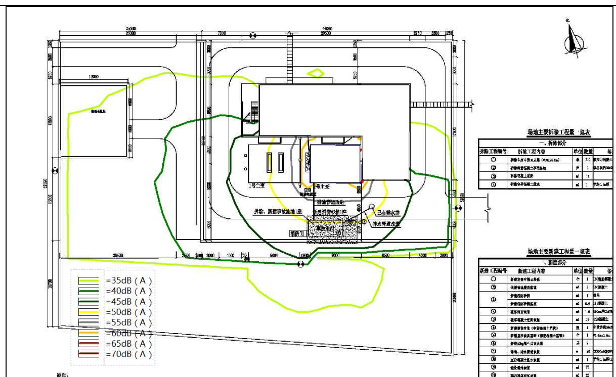
图 9 坚固 110kV 变电站本期规模噪声预测等值线图
