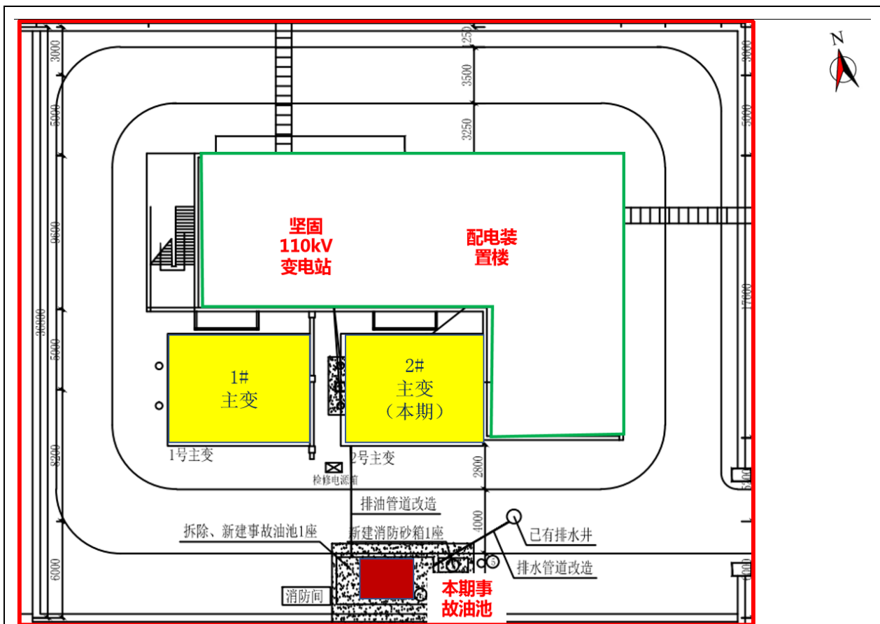
图 2 坚固110kV变电站总平面布置图
