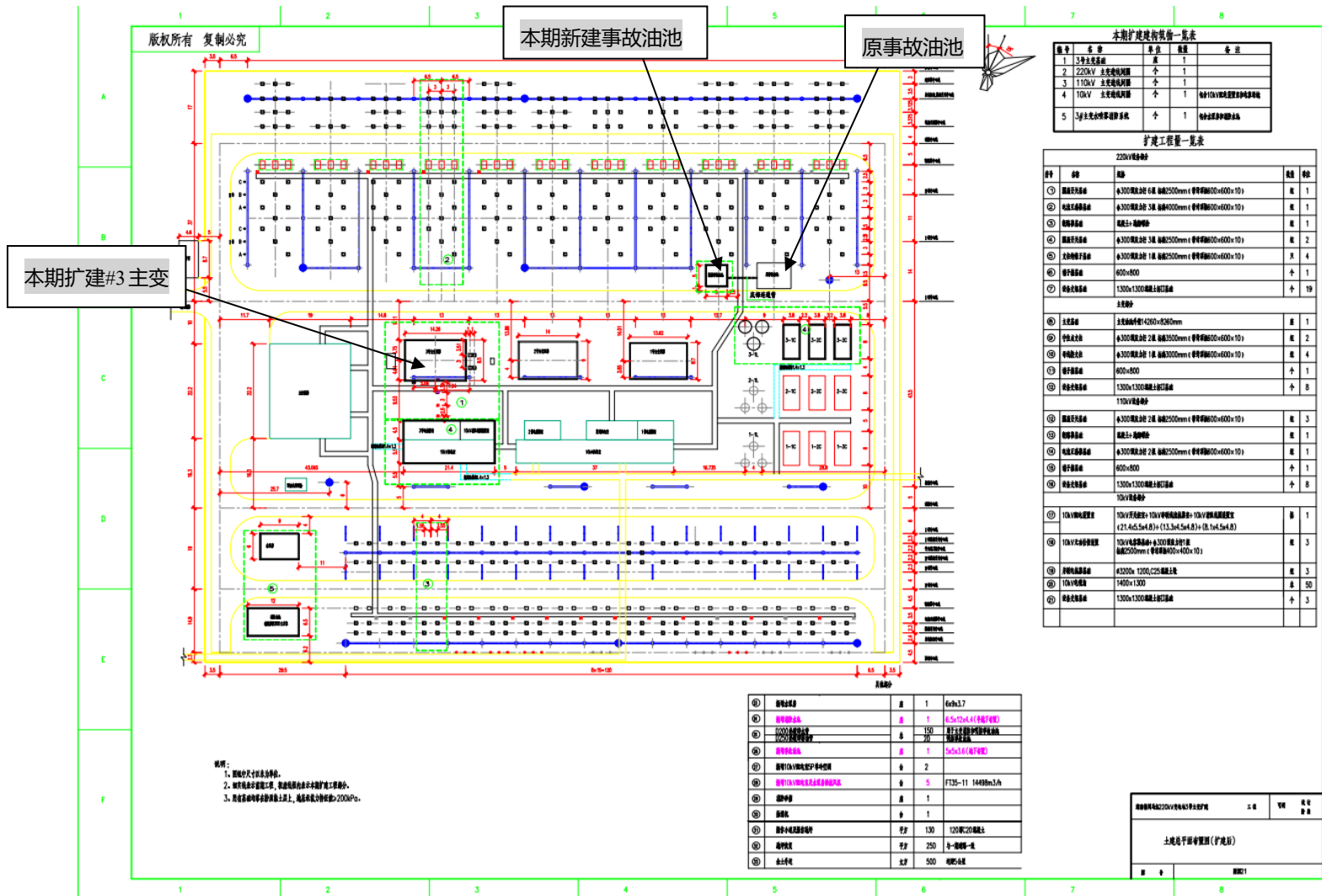
附图 2: 湖南郴州马托 220kV 变电站平面布置图
