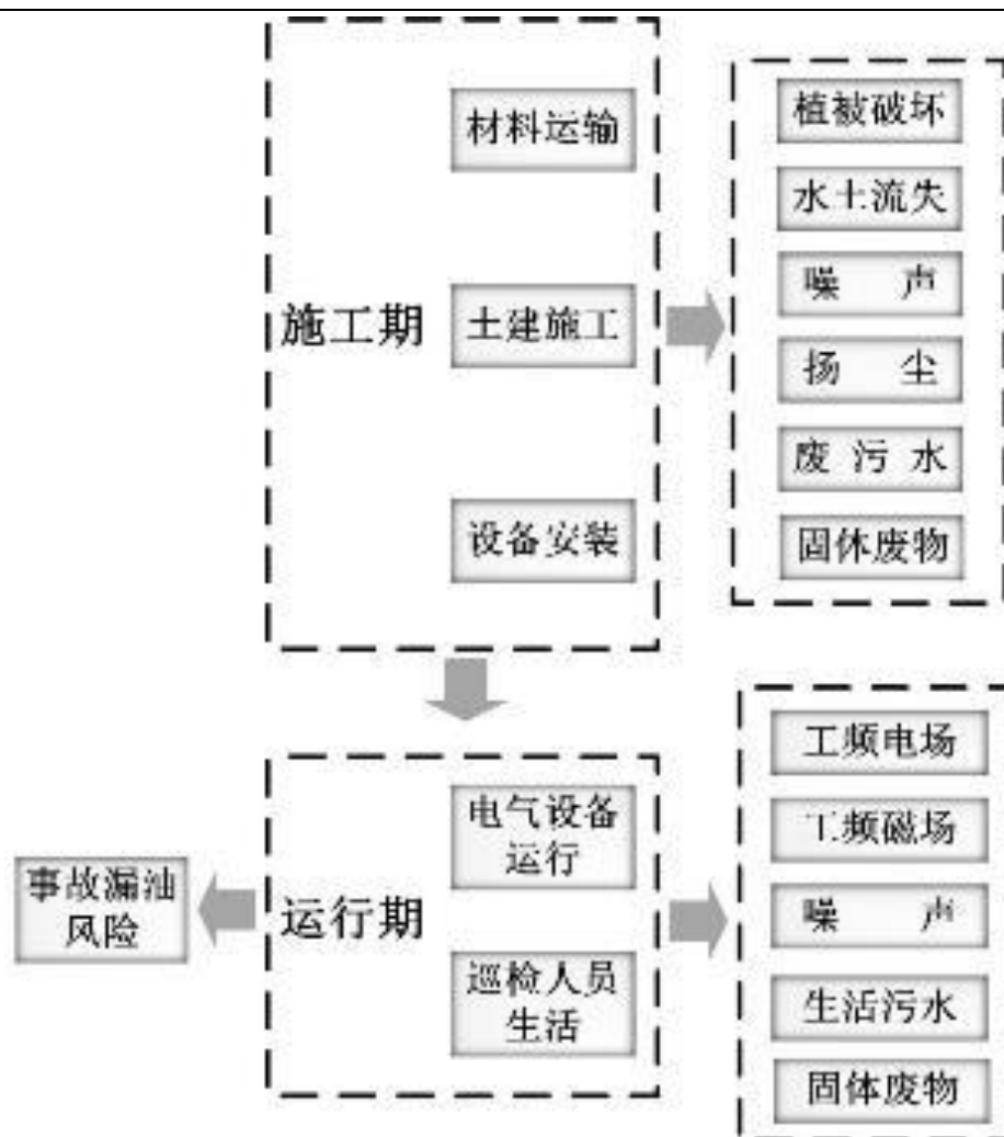
图 2 变电站工程施工期和运行期的产污节点图
