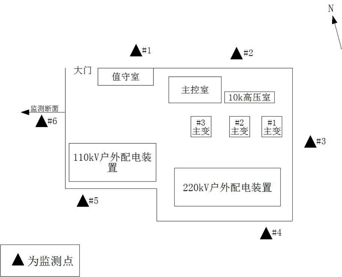
图 1 毛家塘 220kV 变电站平面布置及监测点位示意图
