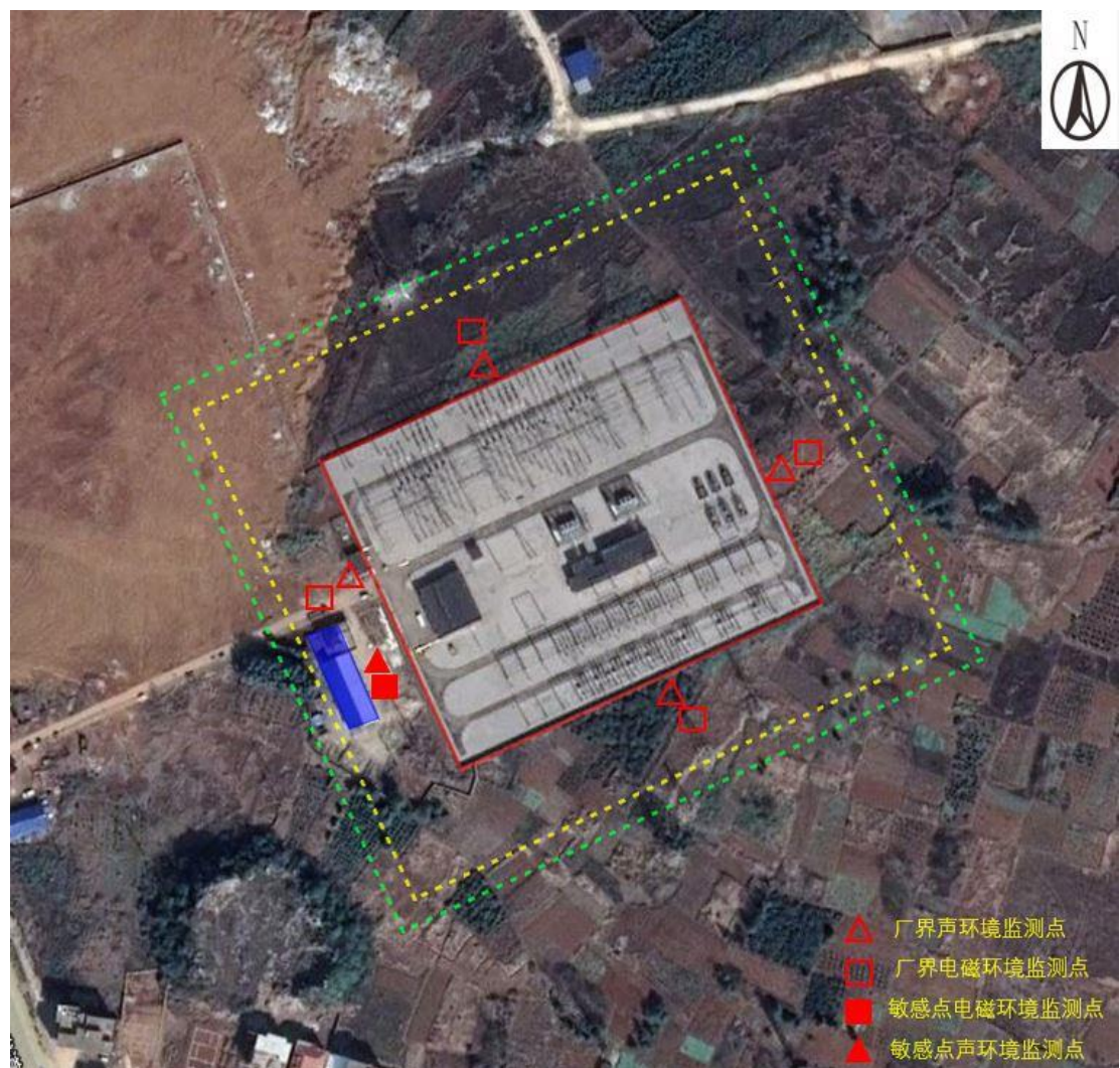
附图 3：湖南郴州马托 220kV 变电站监测布点图
