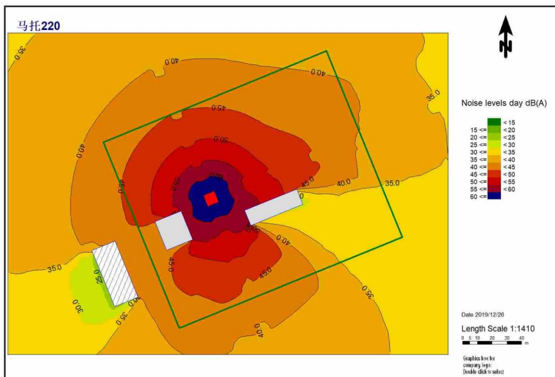
图3 马托220kV变电站本期规模噪声预测等值线图
